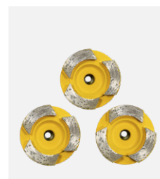
Diamantschijf set voor tegels 3 x Ø 44 mm Artikelnr. 12.328.02
